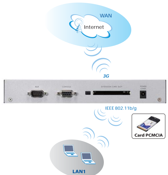
Face arrière ZyWALL USG 100/200
